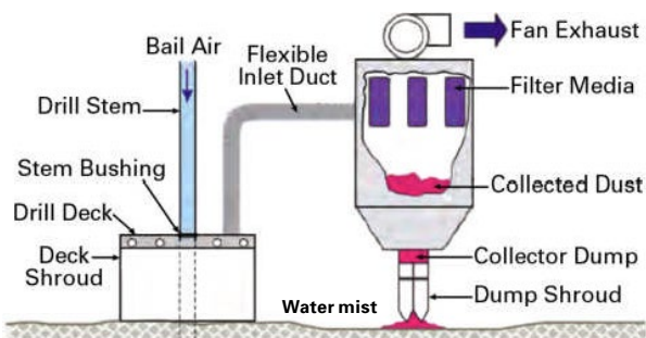
Esquema de los sistemas de eliminación de polvo de los taladros, incluyendo cubiertas para el taladro y la cubierta de descarga.
